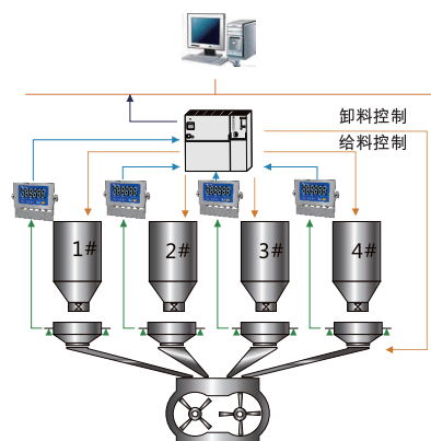
多物料并行配料称重应用
